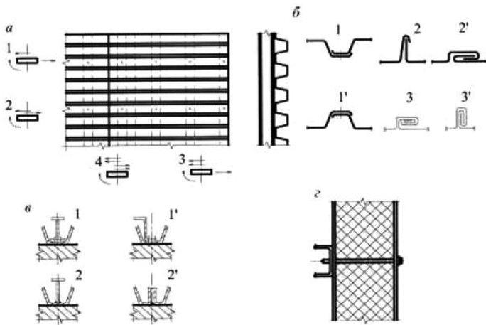
Рисунок 4.1 - Конструктивные формы СМС
