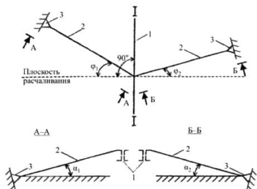
Рисунок К.2 - Схема раскрепления ферм расчалками
